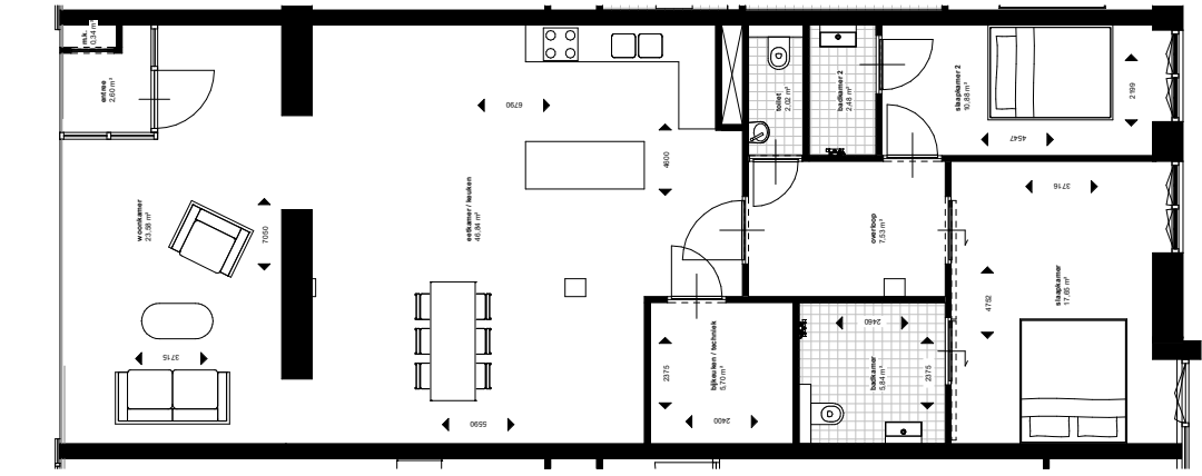
begane grond schaal 1:50
